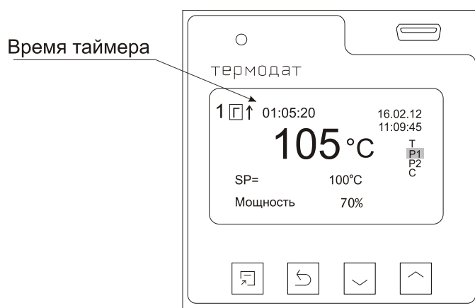
Рисунок 6 – Внешний вид прибора с включенным таймером
