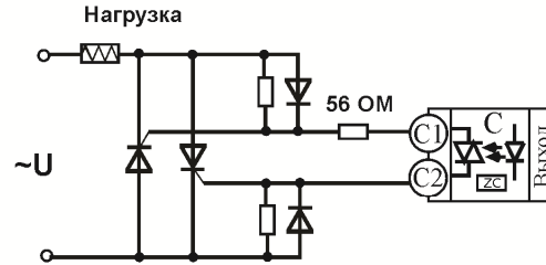
Подключение внешних тиристов
