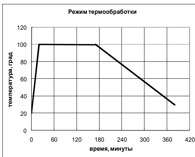
Рисунок 4 –График режима термообработки
