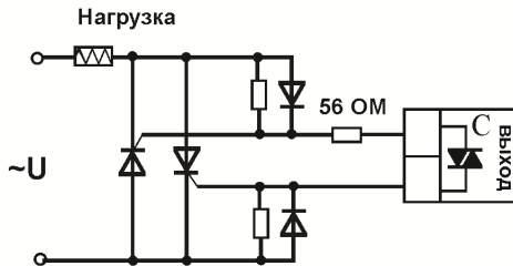
Подключение внешних тиристов
