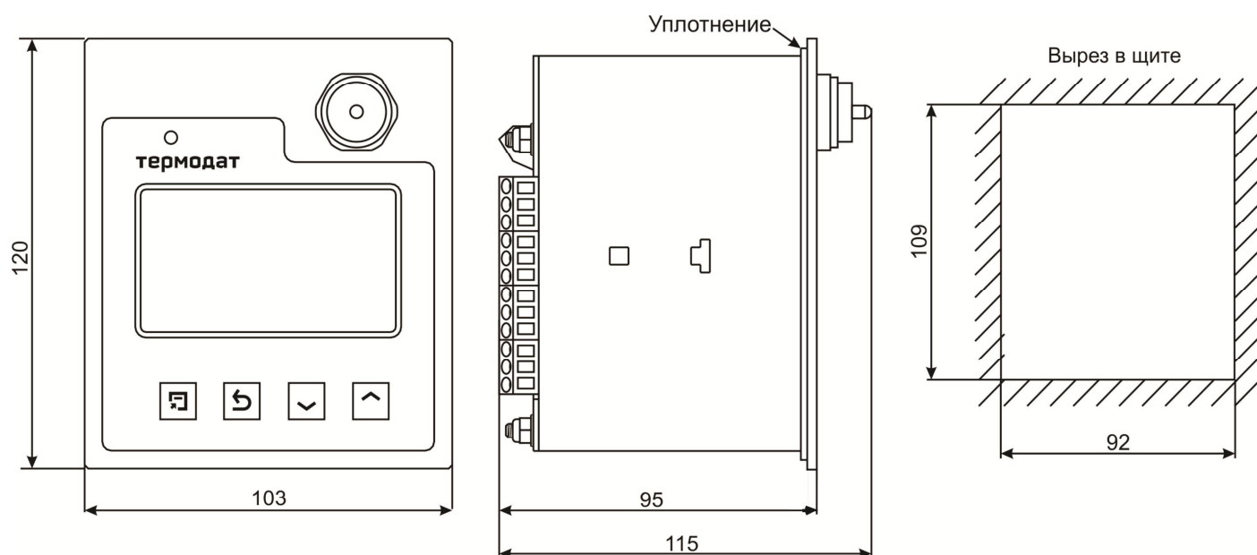
Рисунок 16 – Габаритные размеры прибора Термодат-17Е6/...../F/IP67пп
