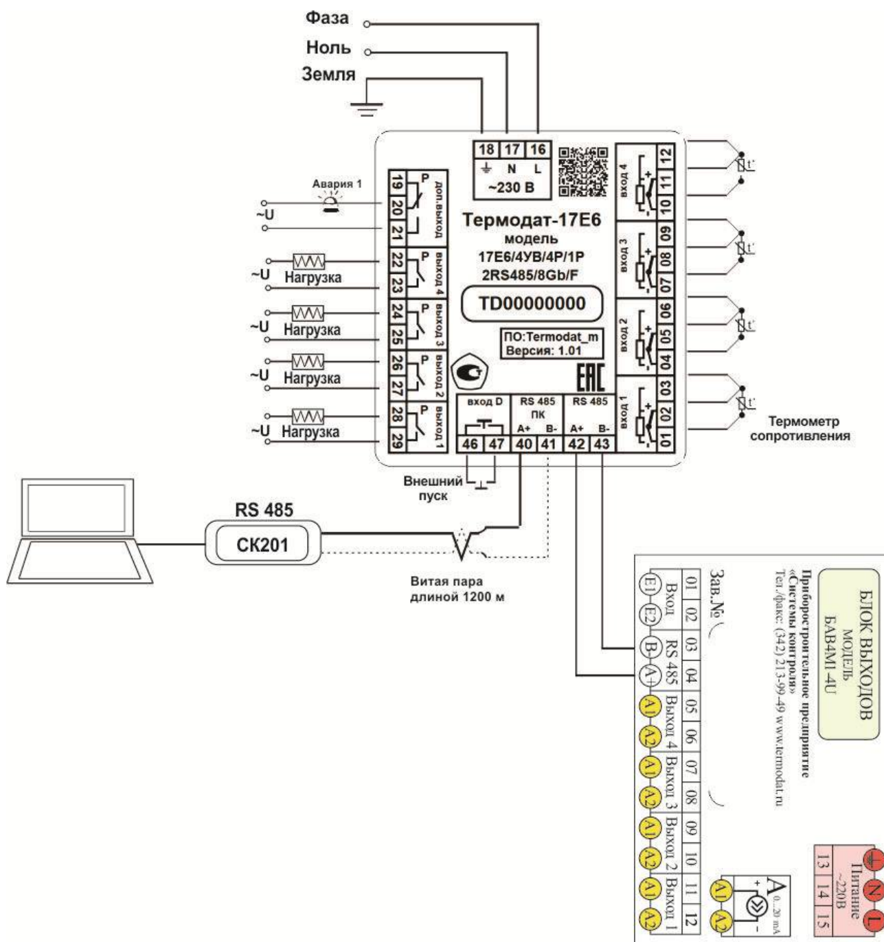
Рисунок 13 – Схема подключения прибора с блоком аналоговых выходов.
